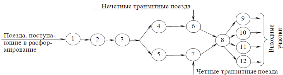
Условные обозначения: 1 – парк приема; 2 – сортировочная горка; 3 – пути сортировочного парка; 4, 5 – вытяжные пути; 6, 7 – приемо-отправочные парки; 8 – подсистема обеспечения локомотивами; 9–12 – прилегающие железнодорожные участки
