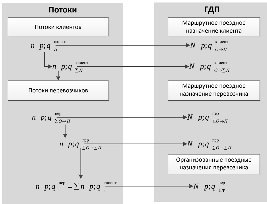
Рисунок 3 – Схема определения способа организации вагонопотоков клиентов в поезда
