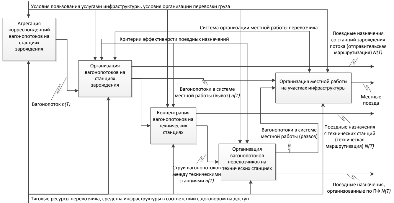
Рисунок 5 – Процесс интегрирования потоков перевозчиков в ГДП
