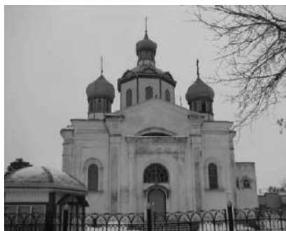
Рисунок 2 – Общий вид здания храма Покрова Пресвятой Богородицы в г. п. Довск Рогачевского района и фрагменты деревянных конструкций купола малого барабана, поврежденных дереворазрушающими грибами
