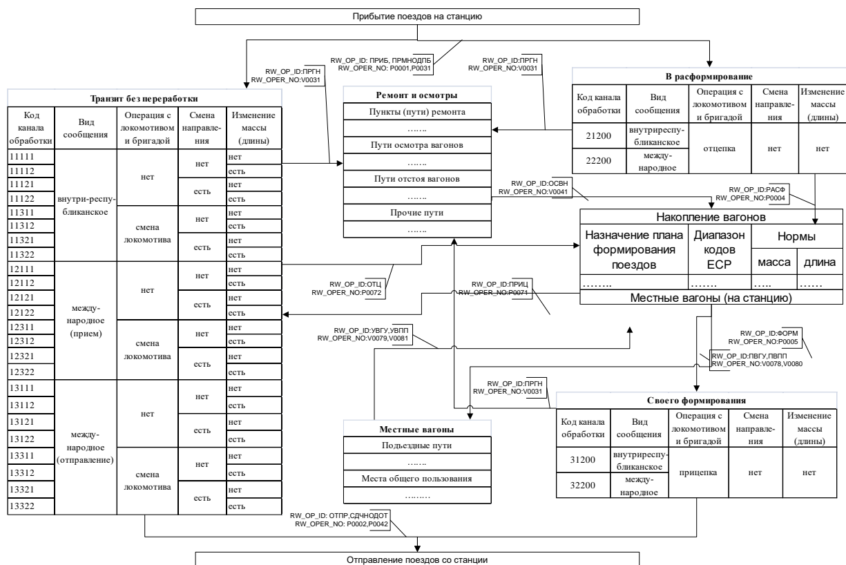
Рисунок 6 – Апостериорная производственная модель УСОГДП
