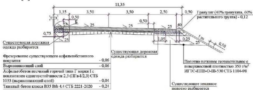
Рисунок 1 – Конструкция дорожной одежды
