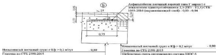
Рисунок 2 – Поперечный разрез разделительной полосы
