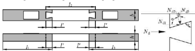
Рисунок 1 – Конструкция составной деревянной шпалы
