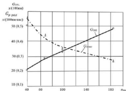
Рисунок 1 – Зависимость расхода топлива G_{100} и удельного расхода топлива на одного пассажира G_{p\ pas} от пассажироместимости исследуемых автобусов
