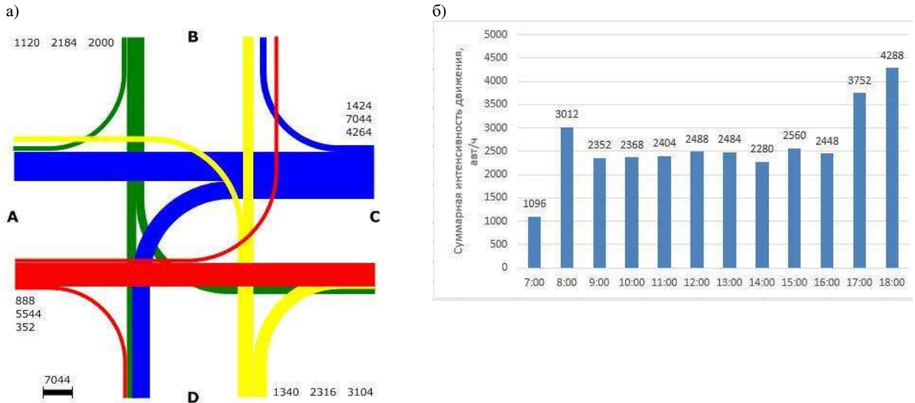
Рисунок 1 – Интенсивности движения на перекрестке ул. Интернациональная – пр-т Ленина: а – цифрограмма интенсивностей (с 07:00 до 19:00); б – интенсивности движения по часам суток
