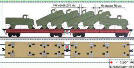
Погрузка порожних грузовых автомобилей в наклонном положении
