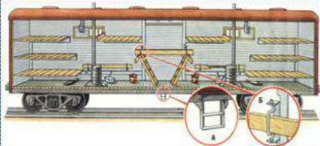
Вагон, оборудованный для перевозки личного состава воинского эшелона
